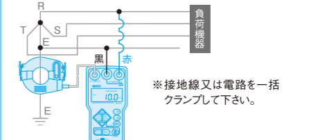
⑤ ACサーボモータの場合 結線モード:1φ/Ior
