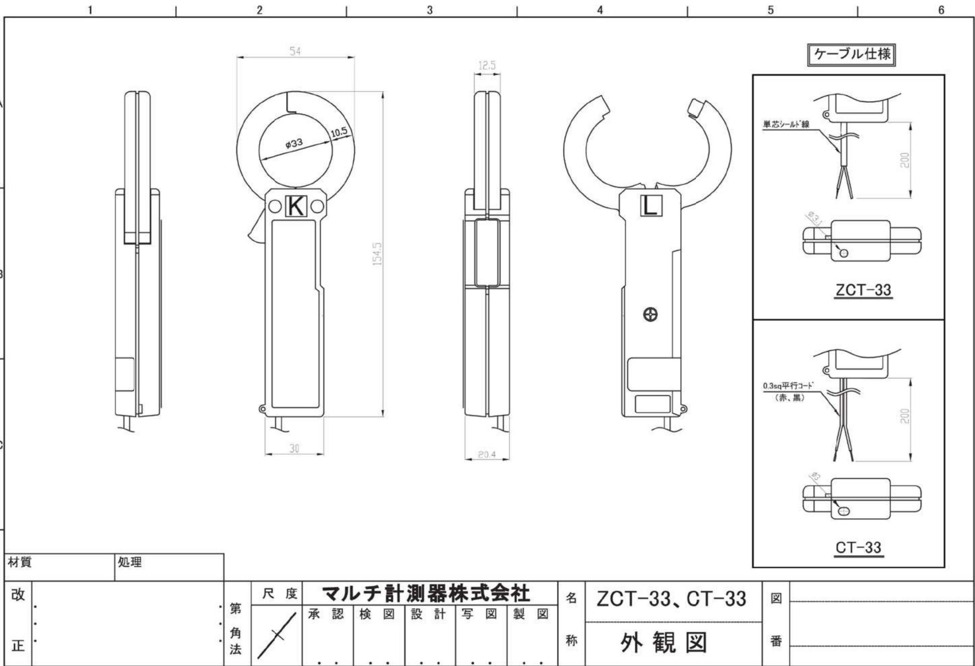
6. 外觀図 (External view) :ZCT-33
