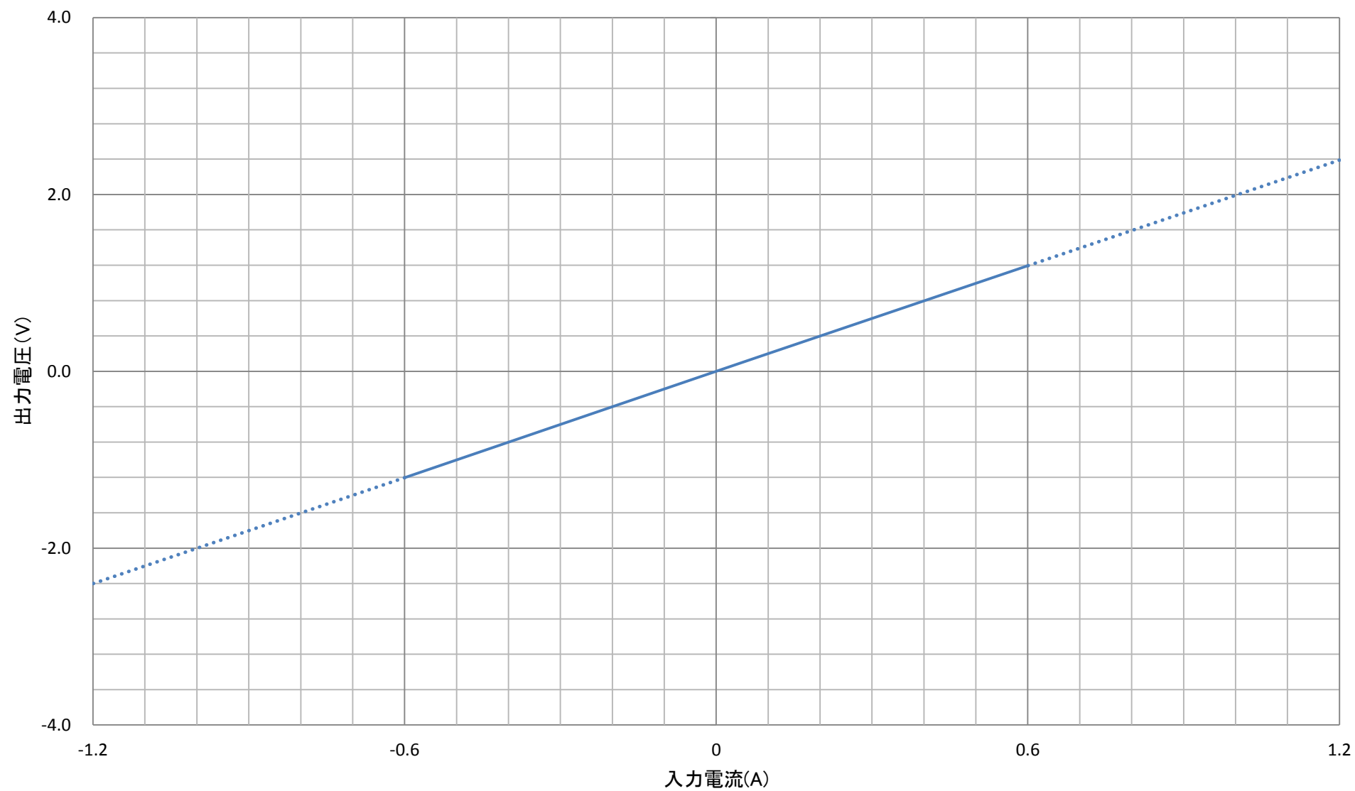
出力特性データ FDAZCT-20L-0.6
