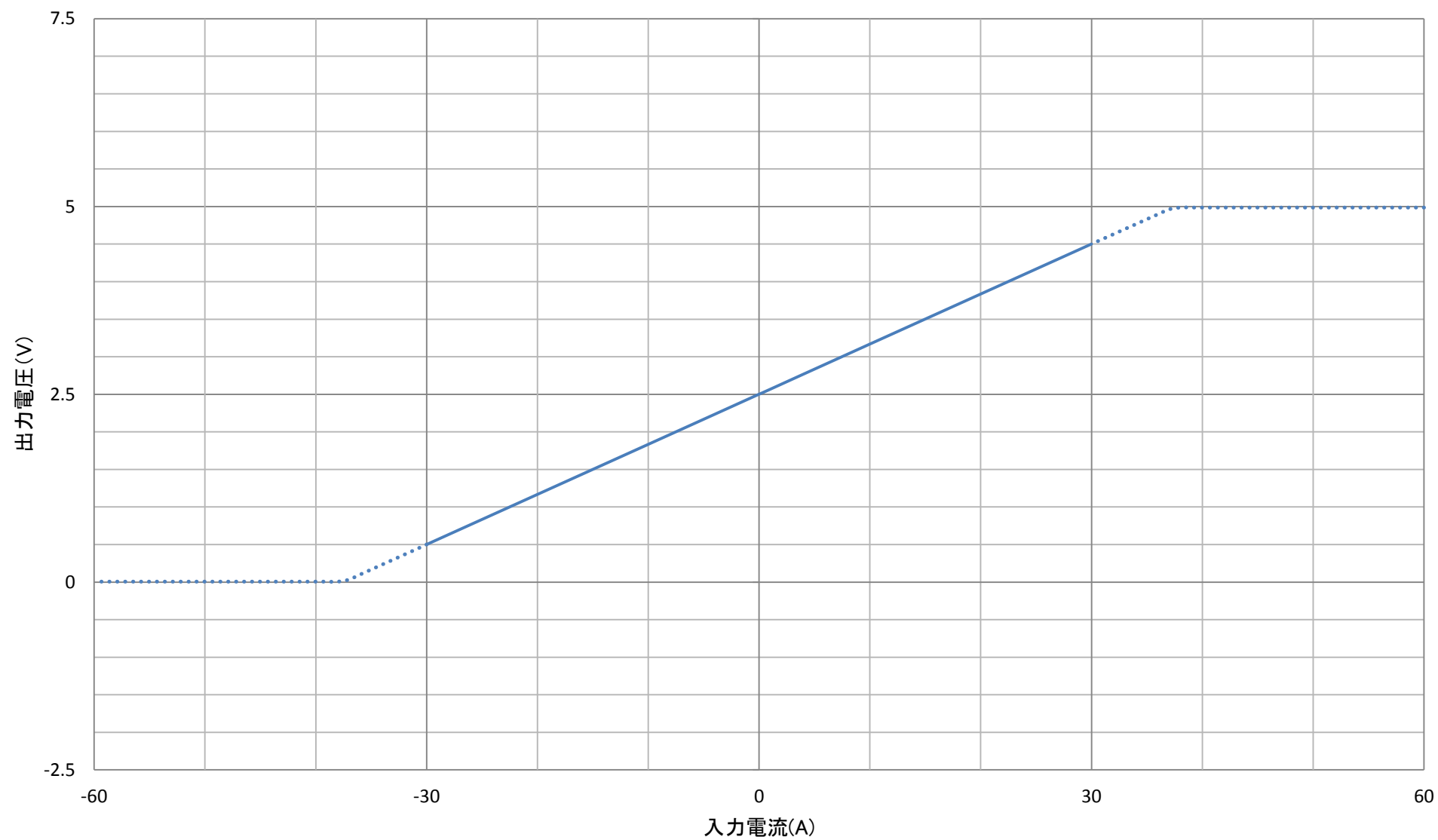
出力特性データ CTF-30-10DC
